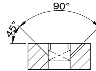
断面図 A-A スケール 1 : 1
