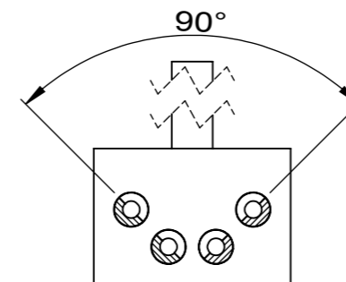
断面図 A-A スケール 1 : 1
