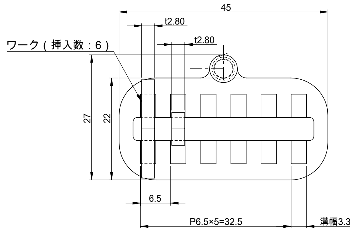
断面図 B-B スケール 2 : 1
