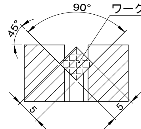
断面図 B-B スケール 2 : 1
