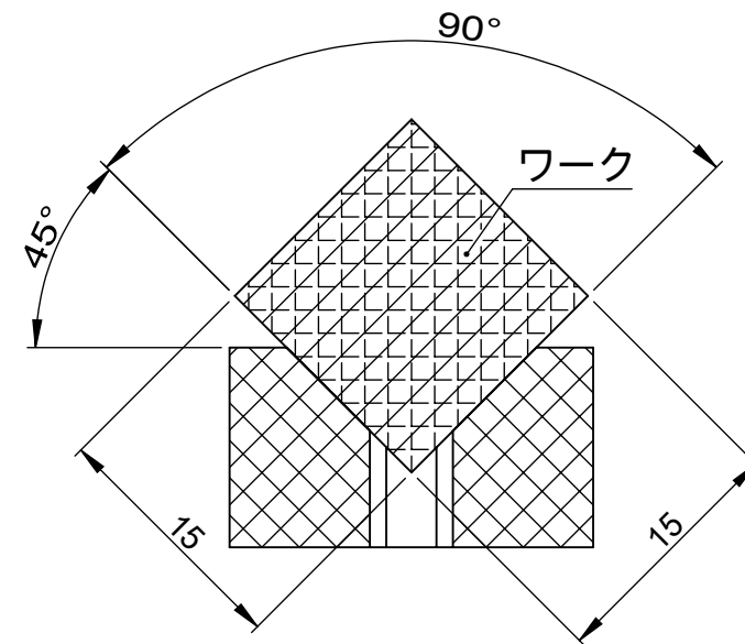
断面図 A-A スケール 2 : 1
