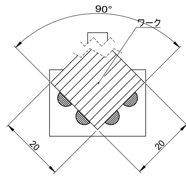
断面図 A-A スケール 1.5 : 1
