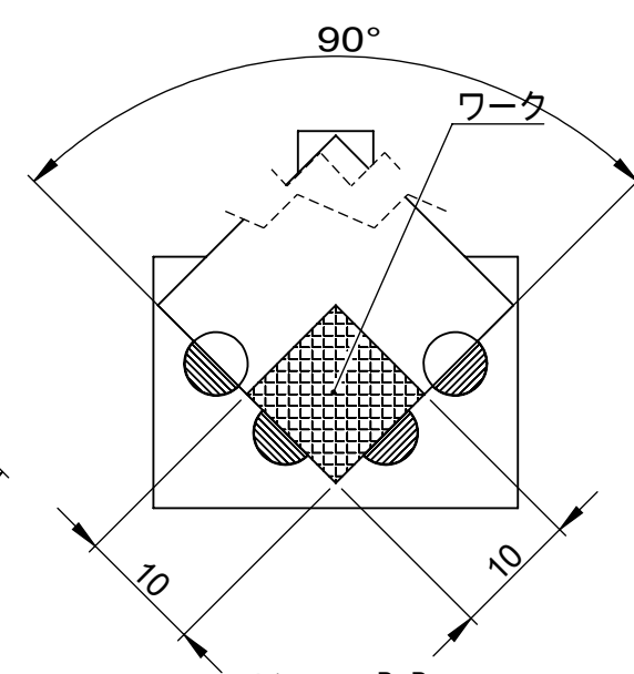
断面図 B-B スケール 1.5 : 1
