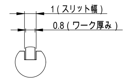
詳細図 C スケール 5 : 1
