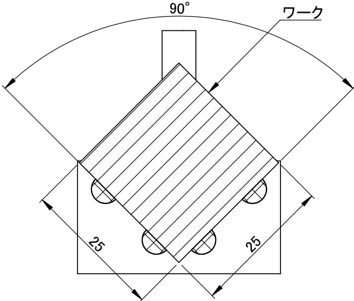
断面図 A-A □25mmワーク収納時
