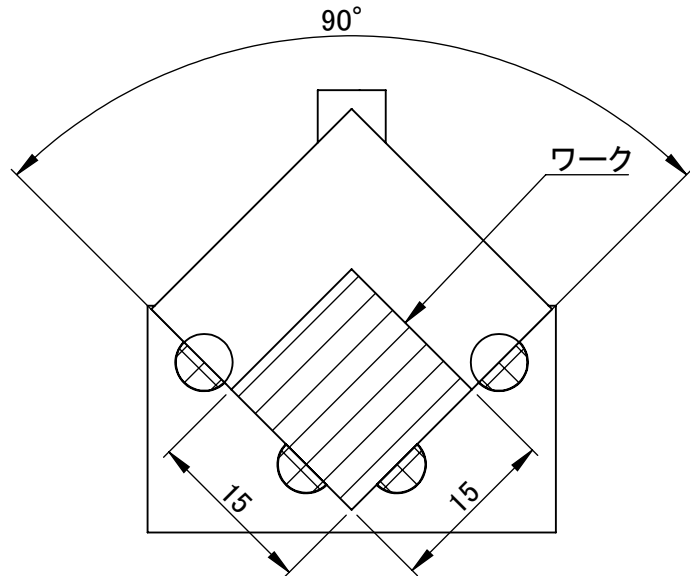
断面図 B-B □15mmワーク収納時
