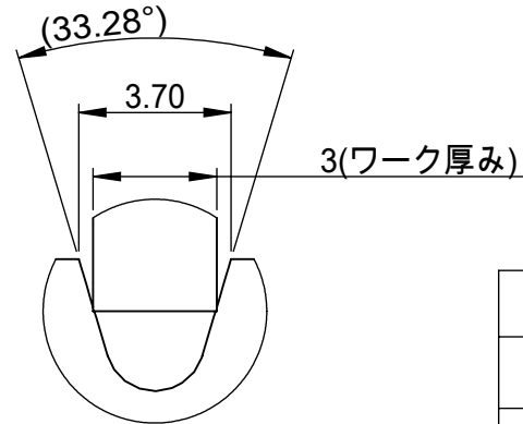
詳細図 B スケール 5 : 1
