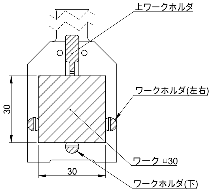
断面図 A-A
