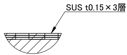
詳細図 B
