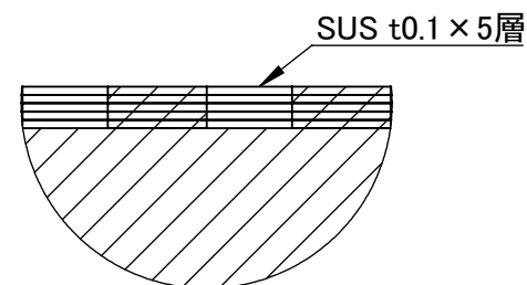
詳細図 B
