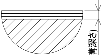
断面図 H-H スケール 1.5 : 1
