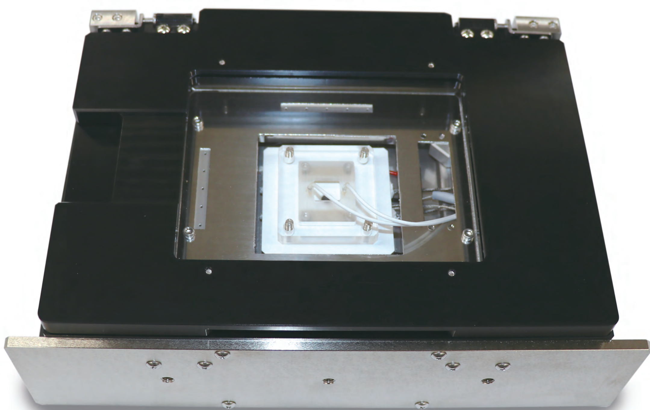
PG1504 温度範囲 -45°C ~ +175°C
